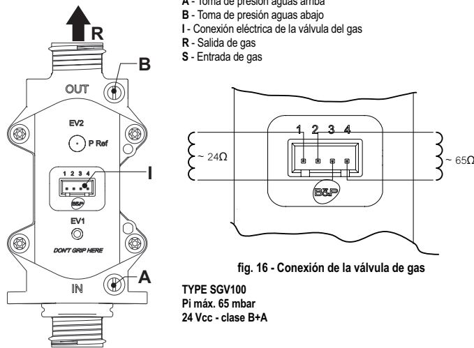
fig. 15 - Válvula del gas
