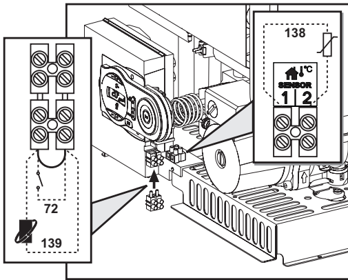
fig. 8 - Acceso a la regleta de conexiones
